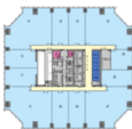
中区平面图
